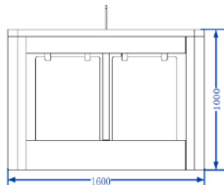
• Vue Frontale
